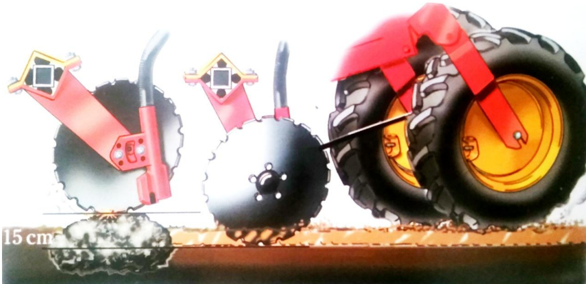
Slika 11: Otpornost na udarac kamena
