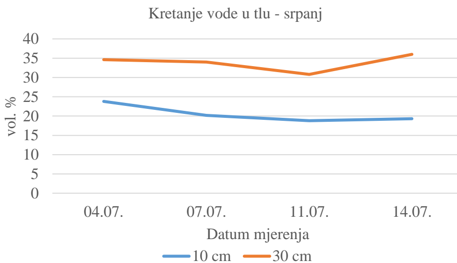
Grafikon 10. Sadržaj vode u tlu izmjeren TDR uređajem tijekom mjeseca srpnja 2017. godine Tijekom prve polovice mjeseca srpnja vrijednosti na 10 cm dubine bile su u rasponu od 23,8 do 23,3 vol. % što je blizu vrijednosti T_v . Odnosno sadržaj vode u tlu na 10 cm dubine bio je toliko nizak da su oštećenja na biljkama ireverzibilna. Prema rezultatima mjerenja na dubini od 30 cm sadržaj vode u tlu bio je u rasponu od 30,8 do 36 vol. % što prema interpretaciji proizvođača predstavlja vrijednost LKV.
