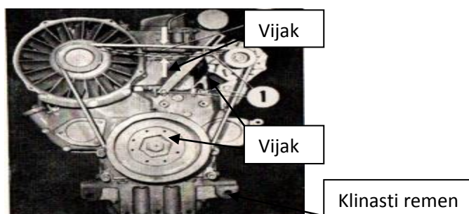
Slika 6. Kontrola zategnutosti klinastog remena
