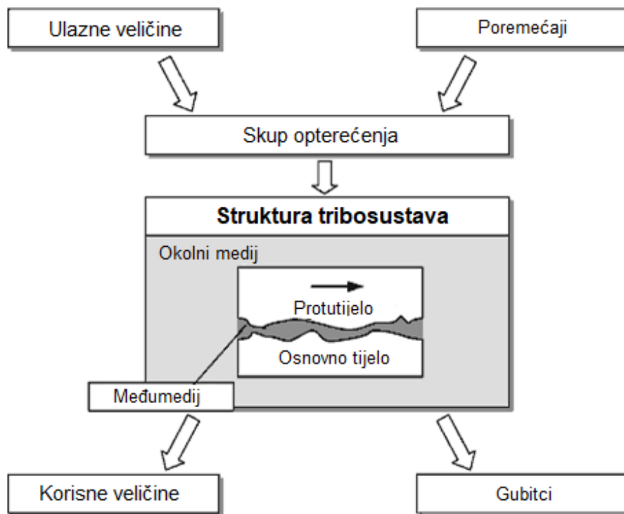
Slika 5. Struktura tribosustava
