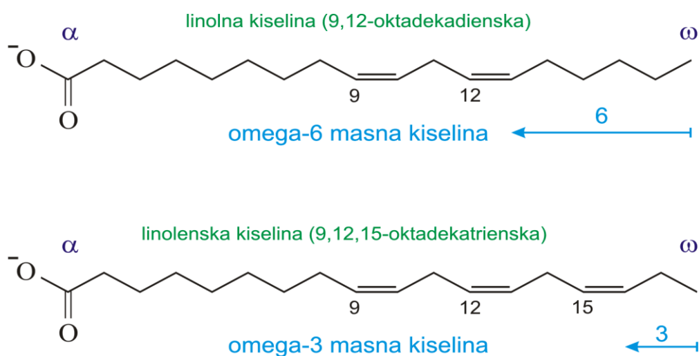
Slika 3. Kemijska struktura Omega-6 i Omega-3 masne kiseline.
