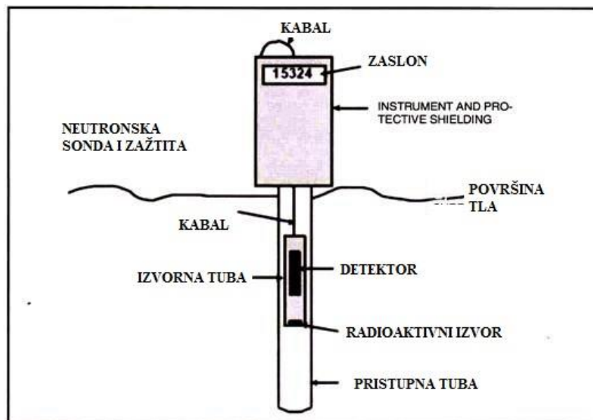
Slika 27. Shema neutronске sonde
