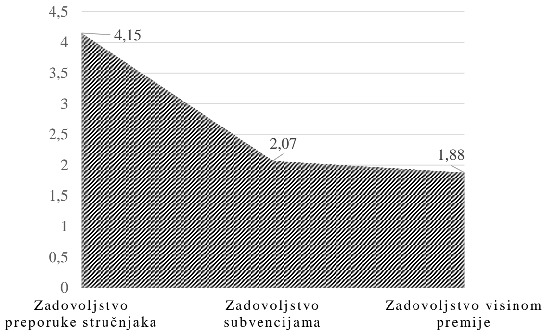
Grafikon 13. Vrednovanje razloga korištenja poljoprivrednog osiguranja
