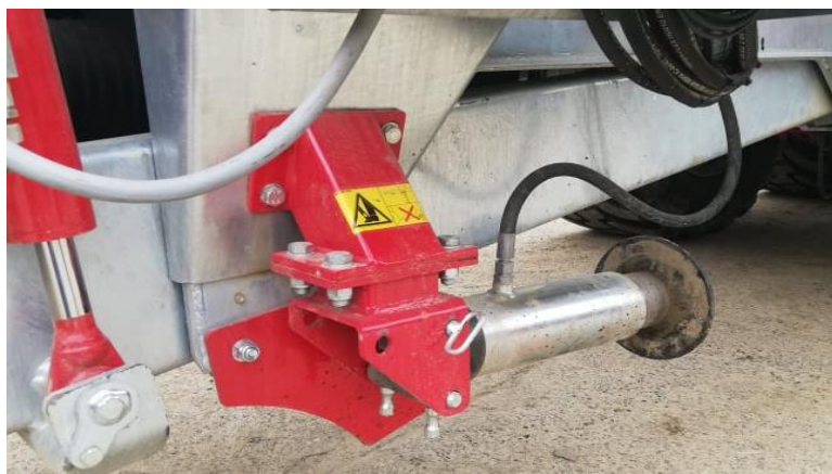
Slika 13. Potporni stup na cisterni Peecon Euroline (Izvor: Kolak, 2020.)
