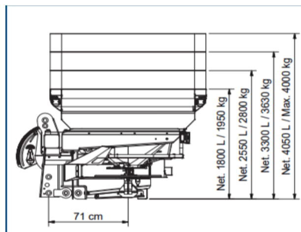
Slika 8. Obujam raspodjelivača Bogballe
