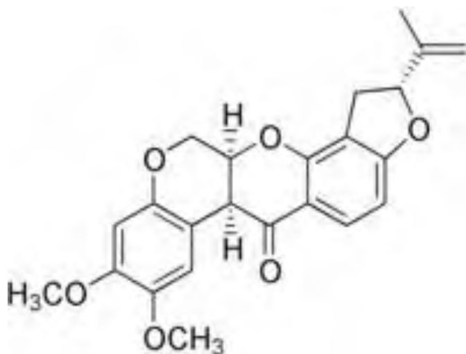
Slika 7. Rotenon molekula
