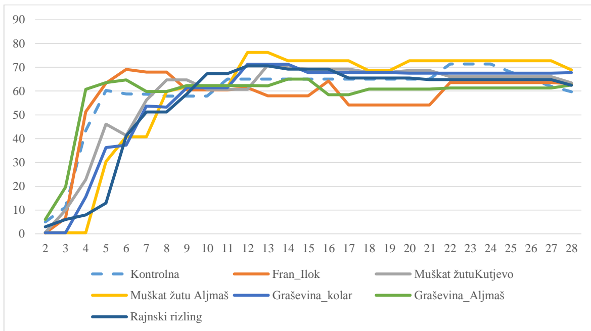
Grafikon 10. Vrijednosti koncentracije metana tijekom anaerobne fermentacije
