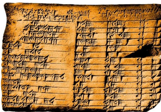
Slika 5. Plimpton 322
