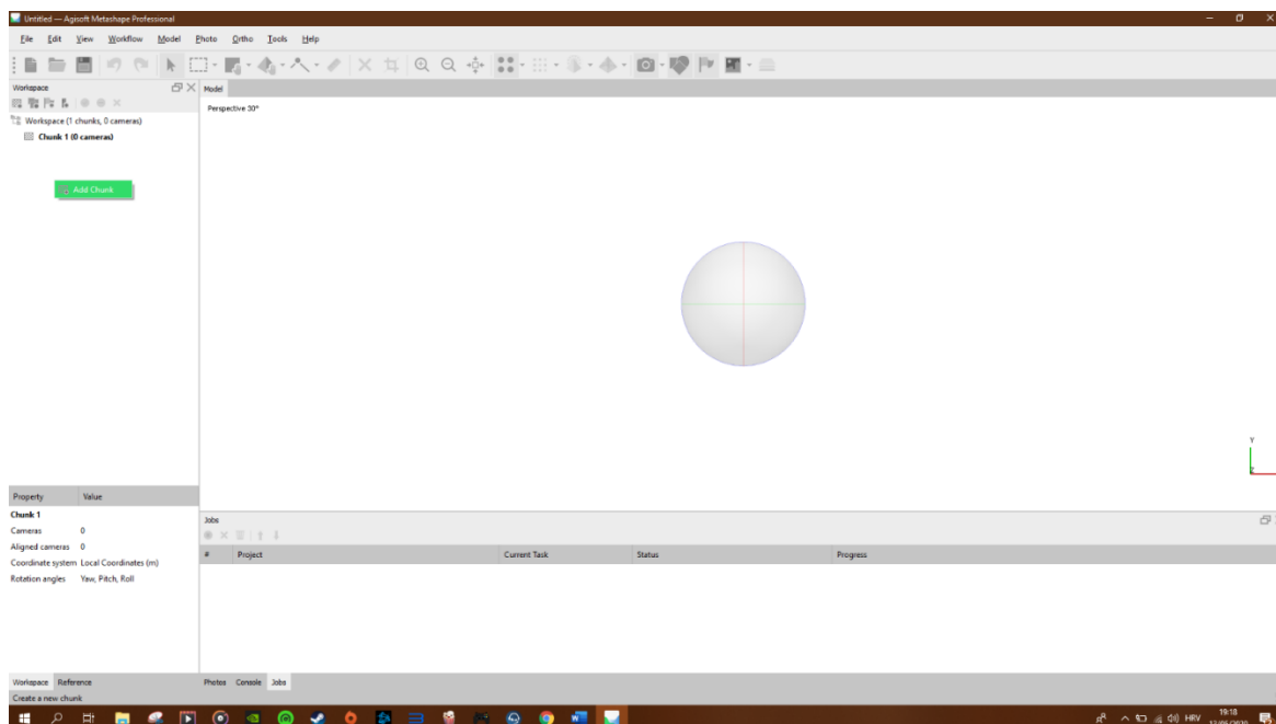
Slika 6. Add Chunk
