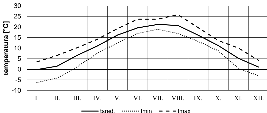
Slika 16. Kretanje srednjih, srednjih minimalnih i srednjih maksimalnih vrijednosti temperature zraka tijekom godine prema mjesečnim podacima na meteorološkoj postaji Slavonski Brod od 1976. do 2005. godine
