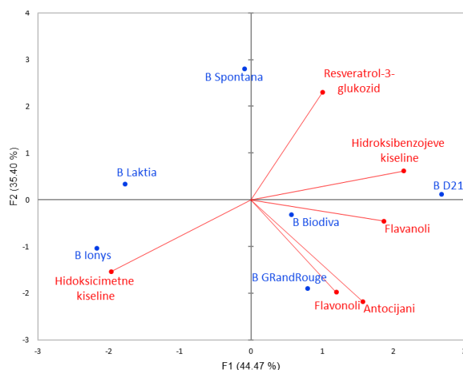
Grafikon 1. Analiza osnovnih komponenti (PCA)- grupe fenolnih spojeva u vinima 'Babić'
