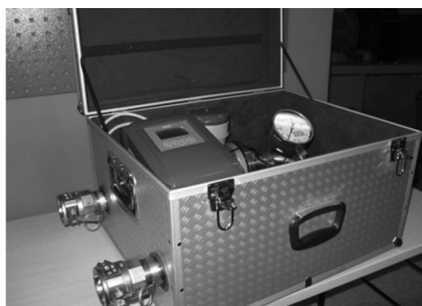
Slika 1. Elektromagnetni mjerač kapaciteta crpke tvrtke Krohne
