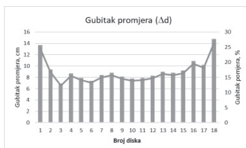
Grafikon 2. Gubici promjera diskova tanjurače uslijed trošenja
