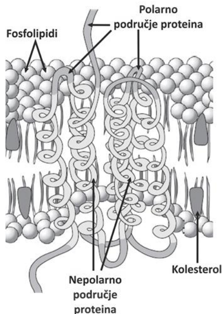
Slika 53. Shematski prikaz građe biomembrane eubakterija i eukariota
