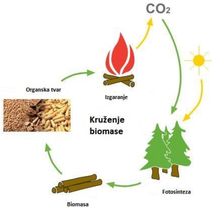
Slika 8. Kruženje biomase
