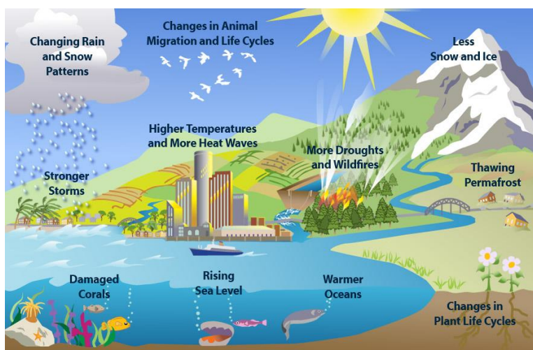
Slika 2. Klimatske promjene
