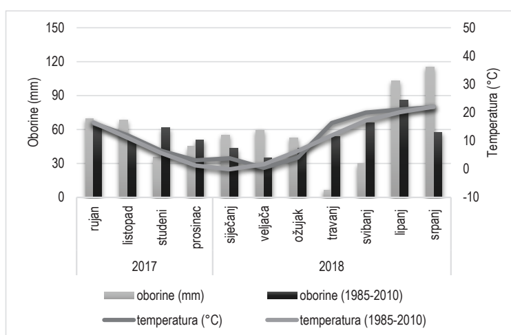
Grafikon 1. Walterov klimatski dijagram za 2017./2018. godinu (1. vegetacijska godina)
