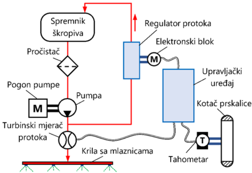
Slika 2. Elektronski regulator (Izvor: vlastita fotografija) Figure 2. Electronic regulator (Source: own photo)
