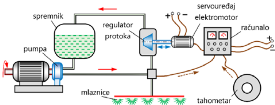
Slika 3. Shema uređaja „Dositron“ (Izvor: vlastita fotografija) Figure 3. Scheme of the "Dositron" device (Source: own photo)
