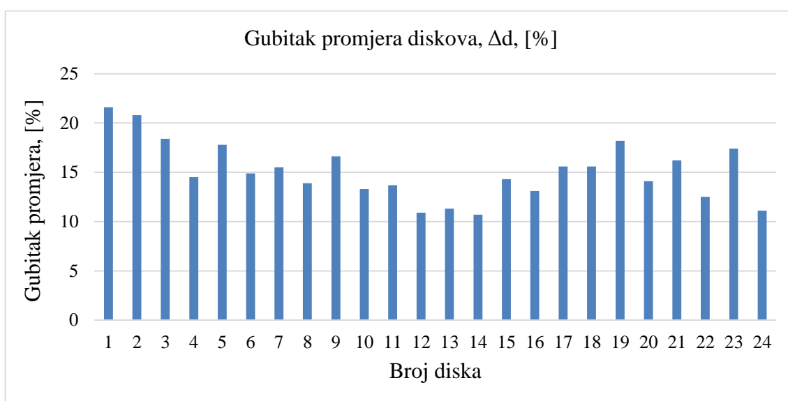
Slika 35. Grafički prikaz smanjenja promjera uslijed trošenja diskova izražen u postocima
