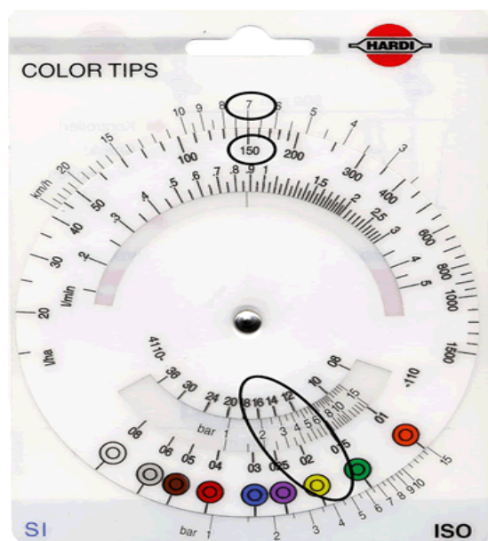
Slika 11. Kalibracijski disk „Hardi“
