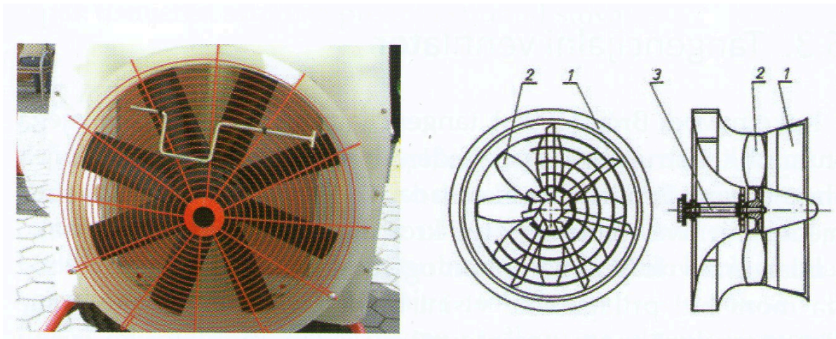
Slika 13. Aksijalni ventilator (1-kućište, 2-lopatice, 3-vratilo ventilatora)
