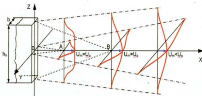
Slika 15. Raspodjela brzina kod pravokutnoga prostornoga mlaza
