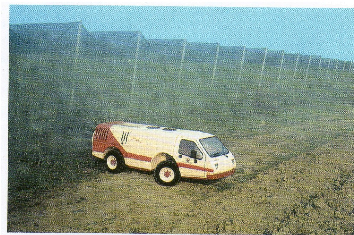
Slika 9. Samokretni raspršivač Izvor: Barčić (1995.)
