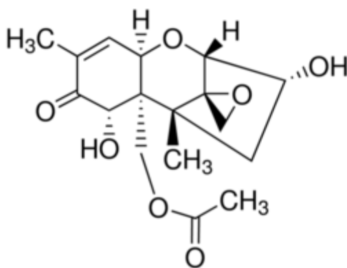
Slika 4. Struktura deoksinivalenola.
