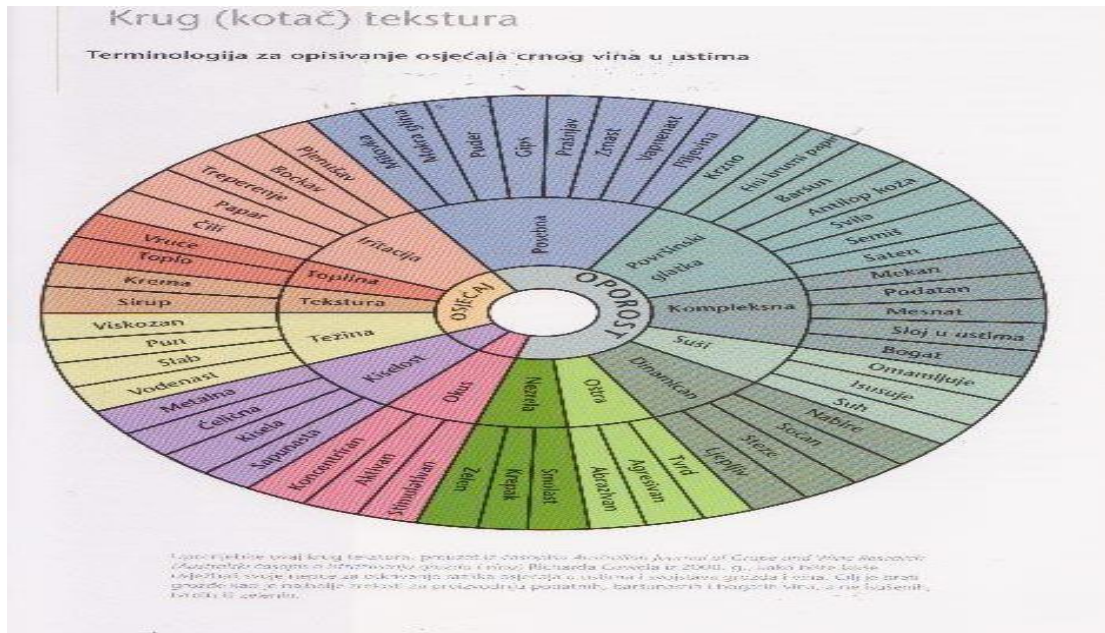
Slika 5. Krug tekstura
