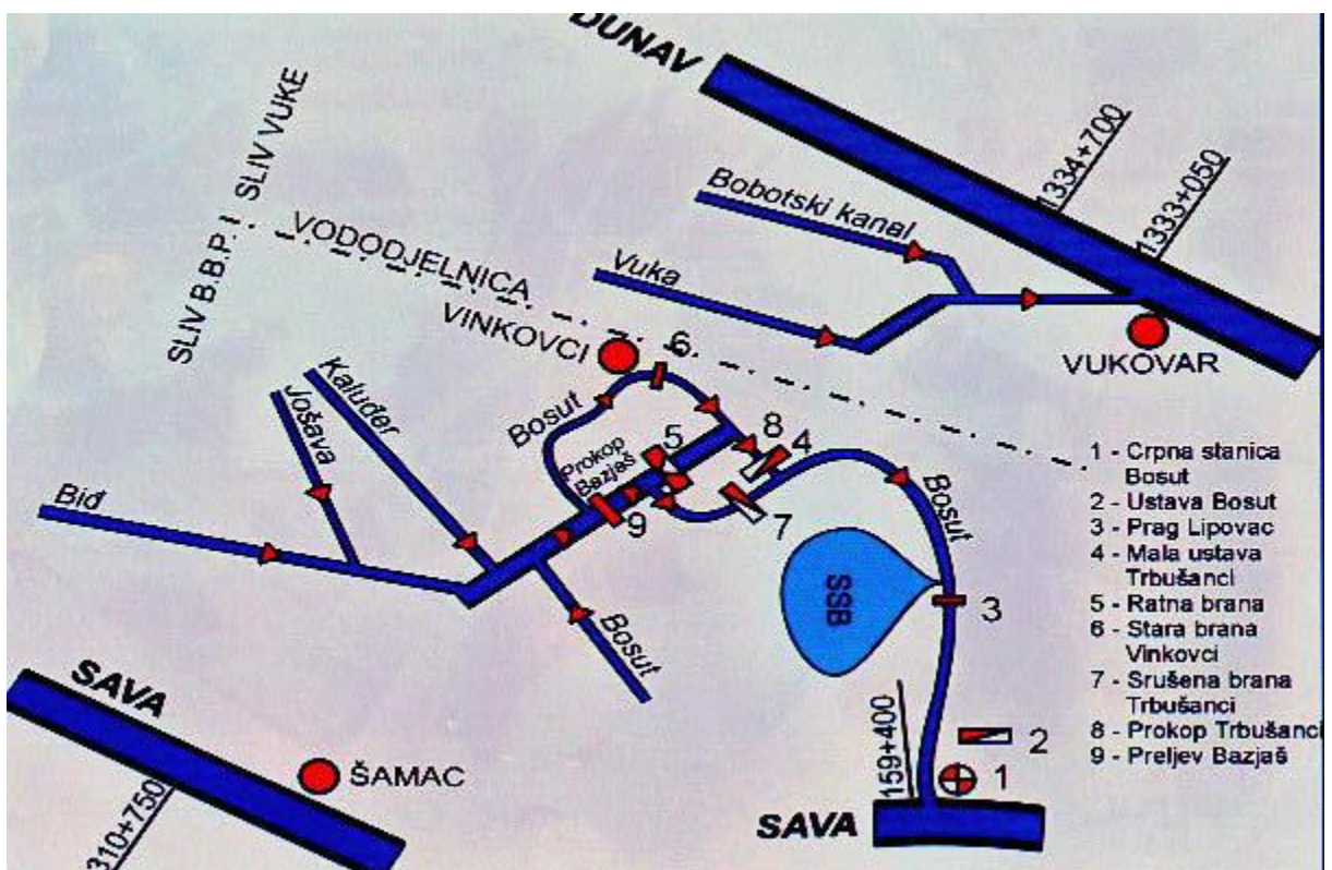
Slika 2. Koncept upravljanja vodama na području Biđ - bosutskog polja (Izvor: Vodoprivreda Biđ-Bosut, Vinkovci, 2013.)
