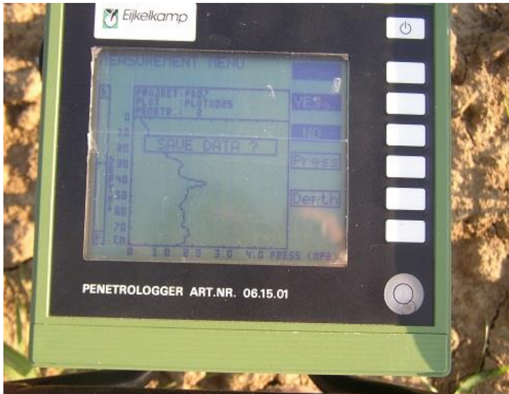
Slika 7. Penetrometar
