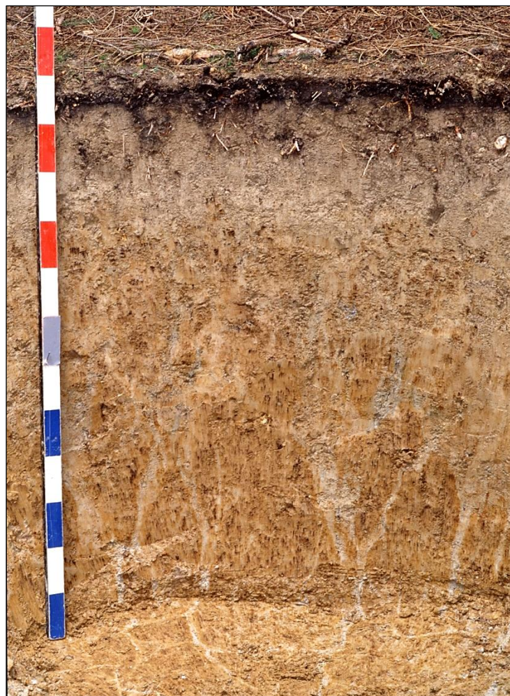
Slika 14. Profil pseudogleja
