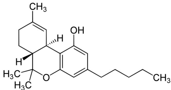
Slika 3. Izgled Tetrahidrokanabinola
