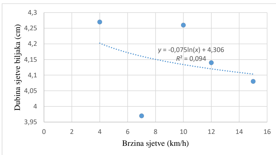
Grafikon 5. Prikaz utjecaja brzine sjetve na ostvarenu dubinu sjetve biljaka
