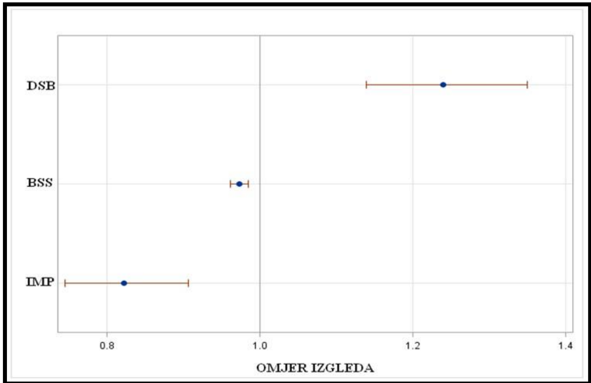
Grafikon 12: Prikaz omjera izgleda s 95% Waldovim intervalom povjerenja za model 1. i kontrolni dan 2. simentalke pasmine)
