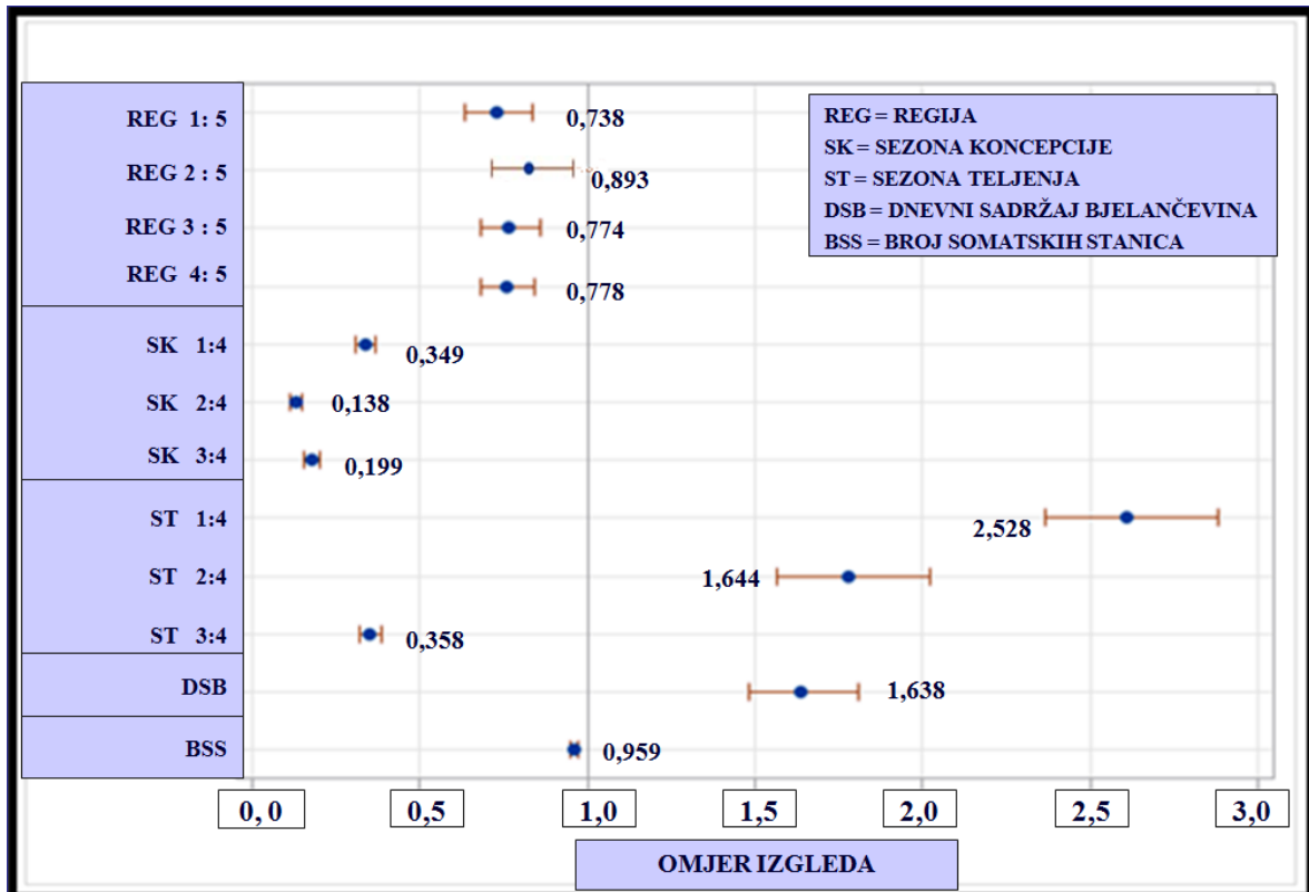
Grafikon 14: Prikaz omjera izgleda s 95% Waldovim intervalom povjerenja za model 2. i kontrolni dan 2. holstein pasmine
