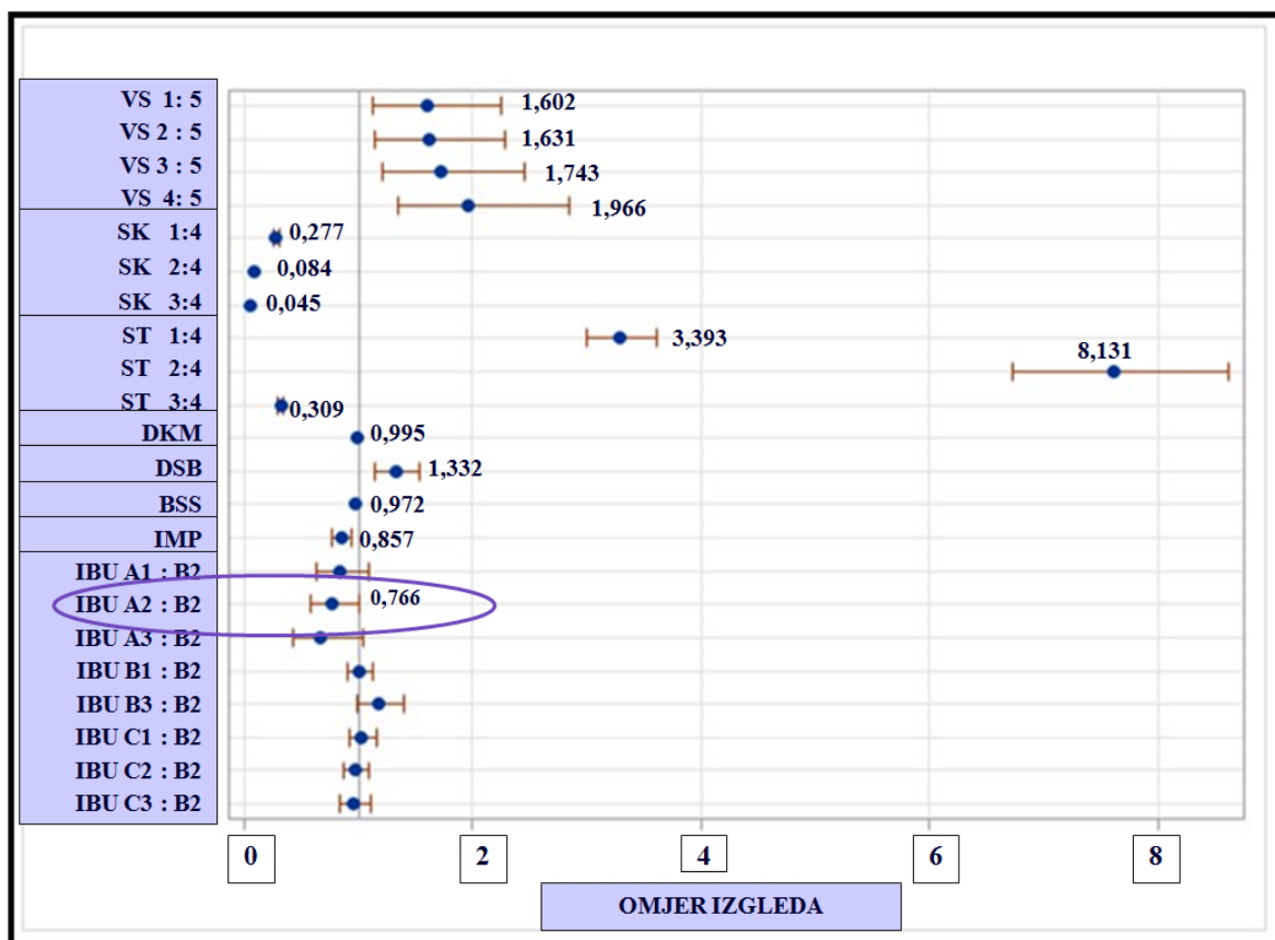
Grafikon 16: Prikaz omjera izgleda s 95% Waldovim intervalom povjerenja za model 2. i kontrolni dan 2. kontrolni dan simentalske pasmine
