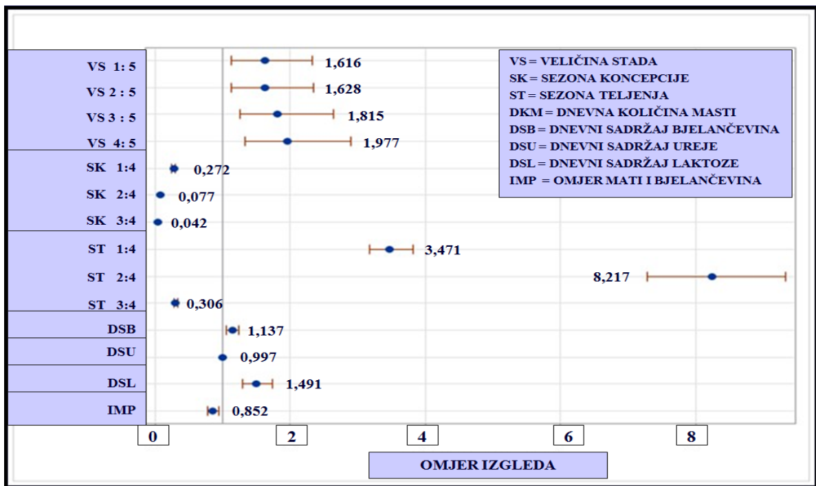
Grafikon 15: Prikaz omjera izgleda s 95% Waldovim intervalom povjerenja za model 2. i kontrolni dan 1. simentalske pasmine
