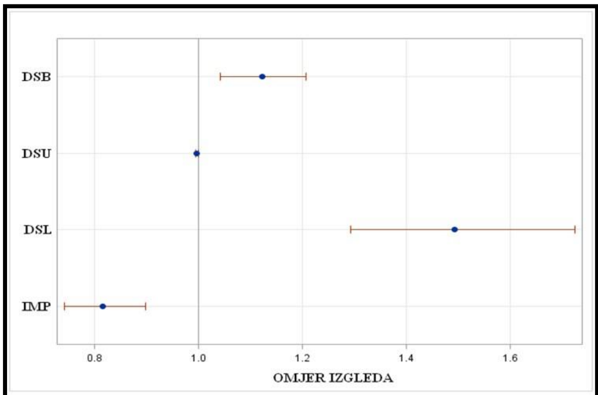
Grafikon 11: Prikaz omjera izgleda s 95% Waldovim intervalom povjerenja za model 1. i kontrolni dan 1. simentalske pasmine
