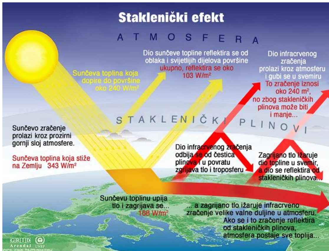
Slika 4. Efekt staklenika
