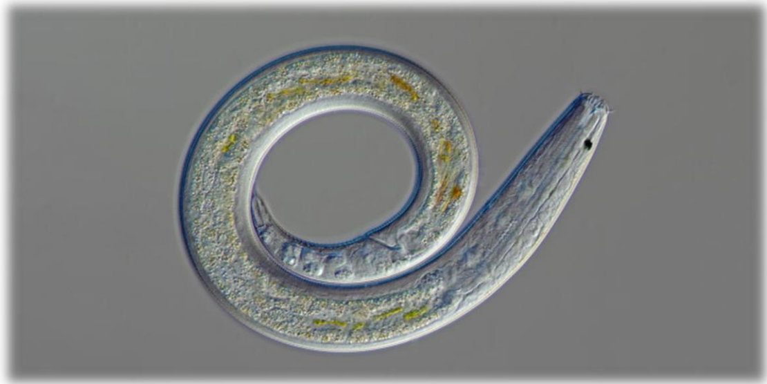
Slika 1. Tijelo nematode
