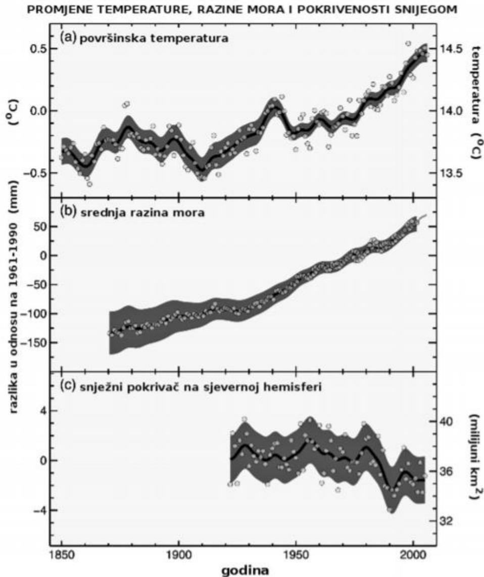
Slika 3. Promjene globalne (a) površinske temperature, (b) srednje razine mora i (c) snježnog pokrivača na sjevernoj hemisferi (Izvor: IPCC, 2007., Branković, 2014.)
