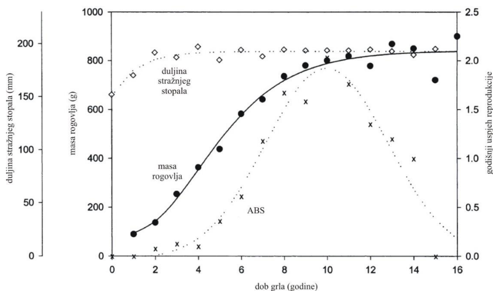
Slika 63. Ovisnost mase rogovlja, duljine stražnjeg stopala i godišnjeg uspjeha reprodukcije o dobi jelena. Izvor: Kruuk i sur, 2002, 1687 p.
