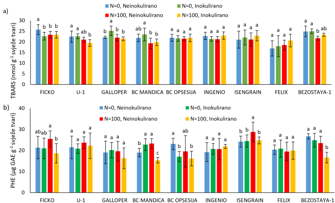
Slika 1. Količina reaktivnih supstanci tiobarbiturne kiseline (TBARS; a) i koncentracija topljivih fenola (PHE; b) u klasovima devet sorti pšenice pri različitim prihranama dušikom (0 kg N ha -1 i 100 kg N ha -1 ) i tretmanom vrstom Fusarium culmorum (neinokulirane i inokulirane biljke). Rezultati su prikazani kao srednja vrijednost šest replika ± standardna devijacija. Različita slova iznad pojedinog stupca označavaju statistički značajne razlike između tretmana unutar svake sorte pojedinačno prema Fisher LSD testu (p ≤ 0,05). Izvor: Matić i sur., 2021a
