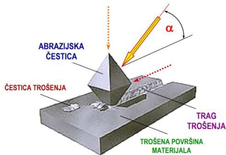
Slika 2. Teorijski model abrazije (Izvor: Heffer, 2002.)
