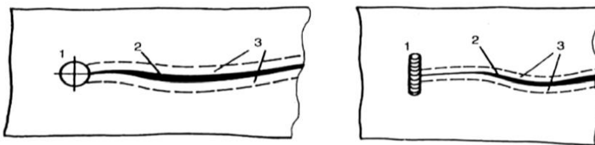
f. Način pripreme spoja za zavarivanje sivog lijeva na hladno 1 – Rupe ili zavari na krajevima pukotine radi sprečavanja njenog širenja; 2 – Pukotina; 3 – Obrada žlijeba
