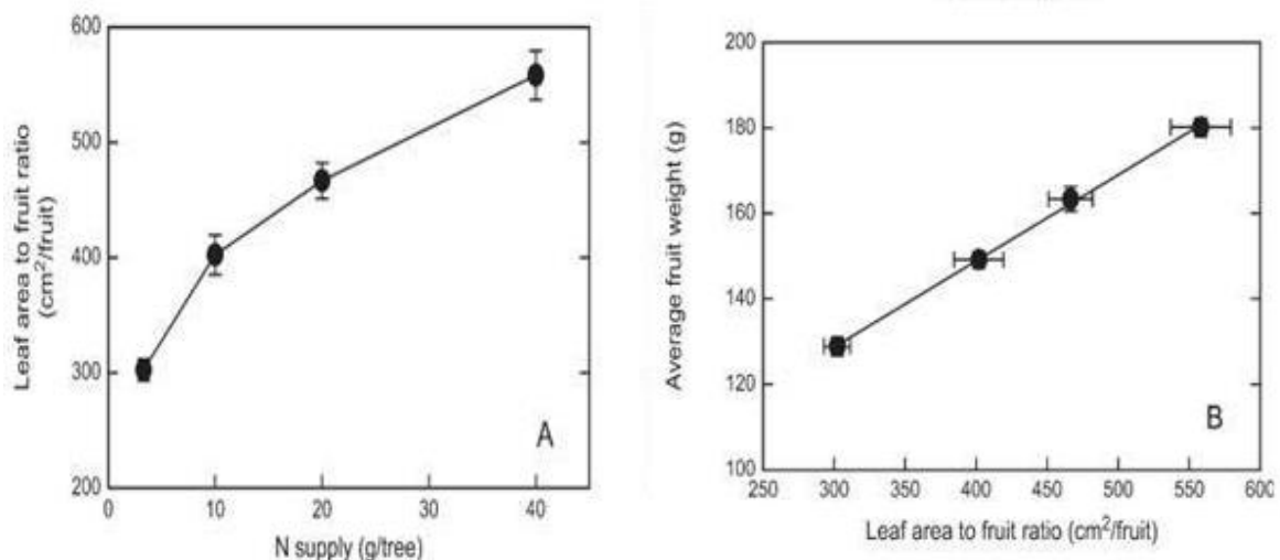
Grafikon 13. A) Reakcija lisne površine u odnosu na opskrbu dušikom i B) Prosječna težina ploda u odnosu na površinu lista (Cheng L., Goffinet M. i Lakso A.) 1
