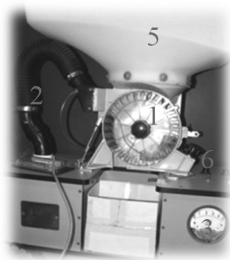
Slika 1. Ispitivana sjetvena sekcija: 1 - sjetveni disk; 2- potisni vod sustava za nadtlak; 3- manometar; 4 - senzor; 5 - sanduk za sjeme; 6 - upravljanje radom sjetvenog diska i ventilatora nadtlaka
