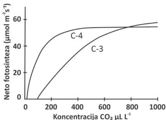
Slika 44. Tipičan intenzitet fotosinteze C-3 i C-4 biljaka u odnosu na koncentraciju CO 2 okoline
