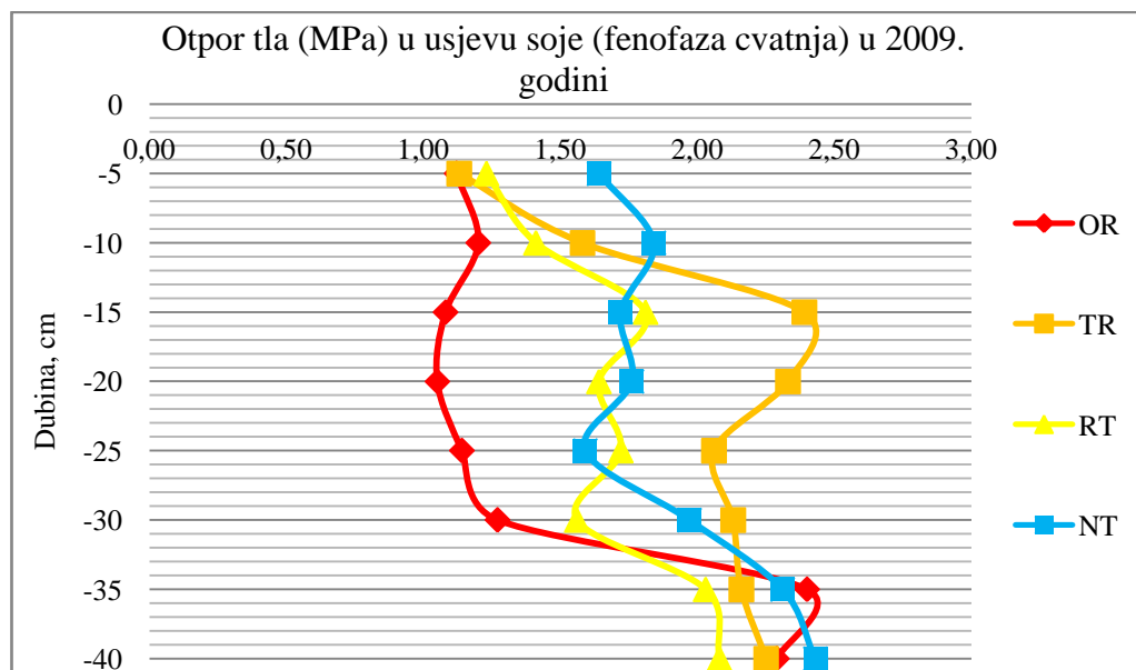
Grafikon 4. Grafički prikaz otpora tla po varijantama obrade tla za soju u 2009. godini (fenofaza cvatnje)
