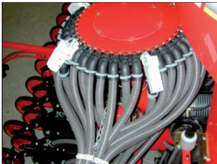
Slika 13. Razvodnik sjemena s magnetnim zaklopkama (Izvor: Uputa za rad, Art.: 80441702 hr)
