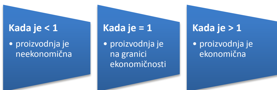
Slika 7. Koeficijent ekonomičnosti
