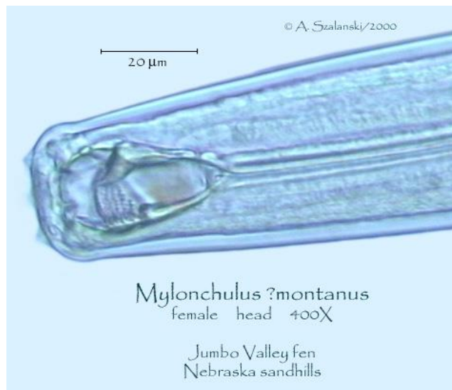
Slika 10. Mylonchulus montanus
