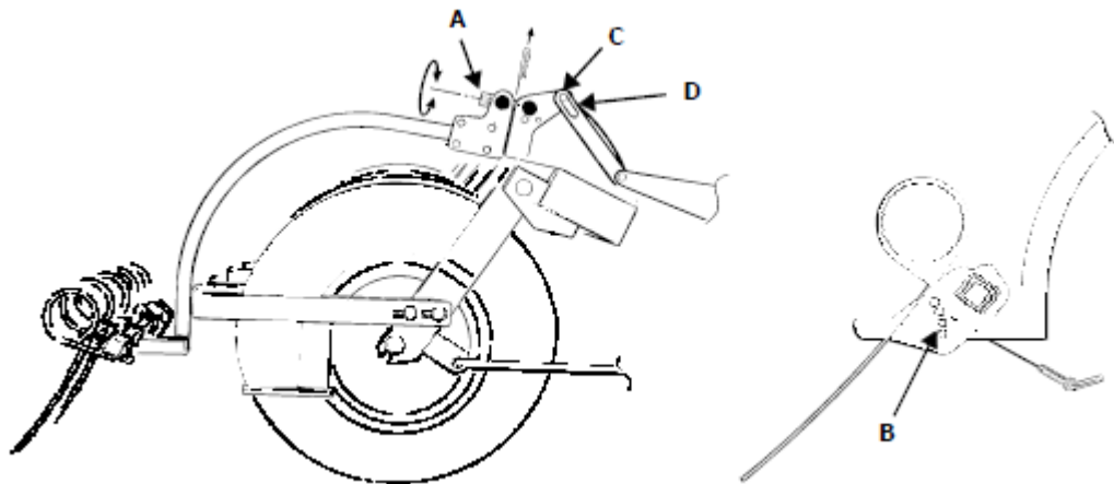
Slika 12: Podešavanje zagrtča
