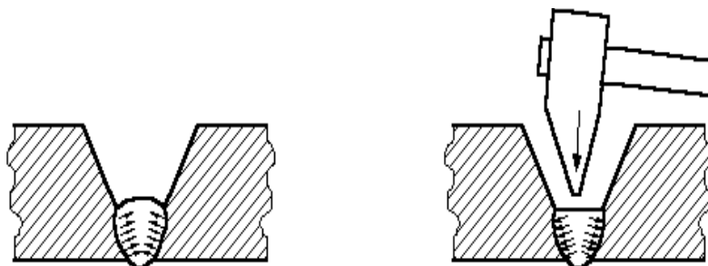
Slika 10. Čekićanjem se smanjuju sile stezanja i smanjuje vjerojatnost pojave pukotina.
