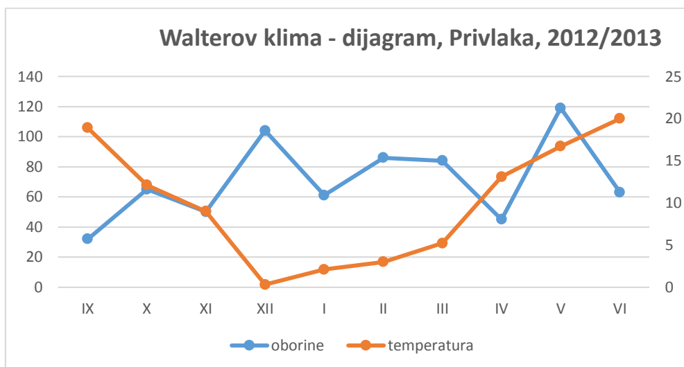
Grafikon 1: Walterov klima-dijagram, Privlaka 2012/2013. (Vlastita mjerenja)
