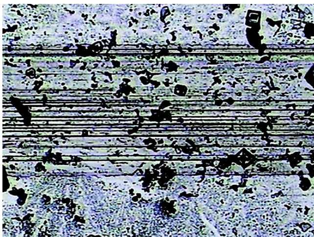
Slika 8. Trošenje tribokorozijom
